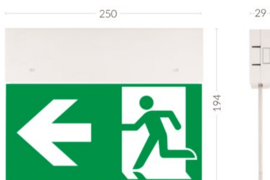
MÅLSKISSE
